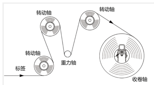
3 利用多重转轴及重力轴相互配合，达到标签回转的效果
